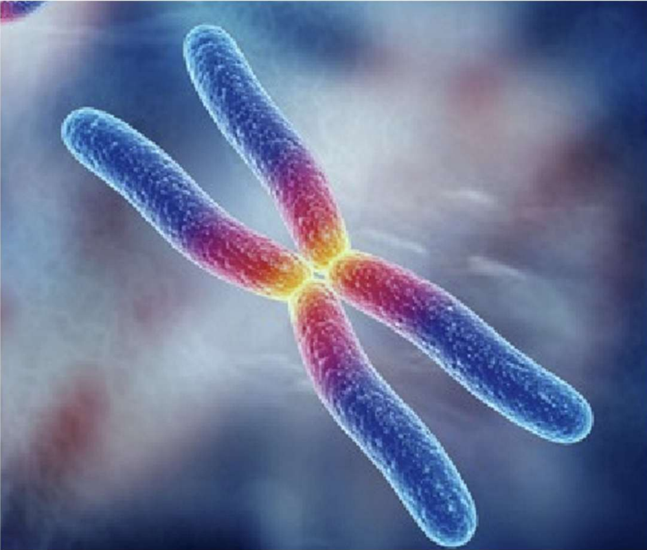
Chromosom
